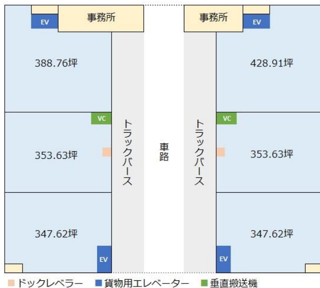
【1階平面図】
