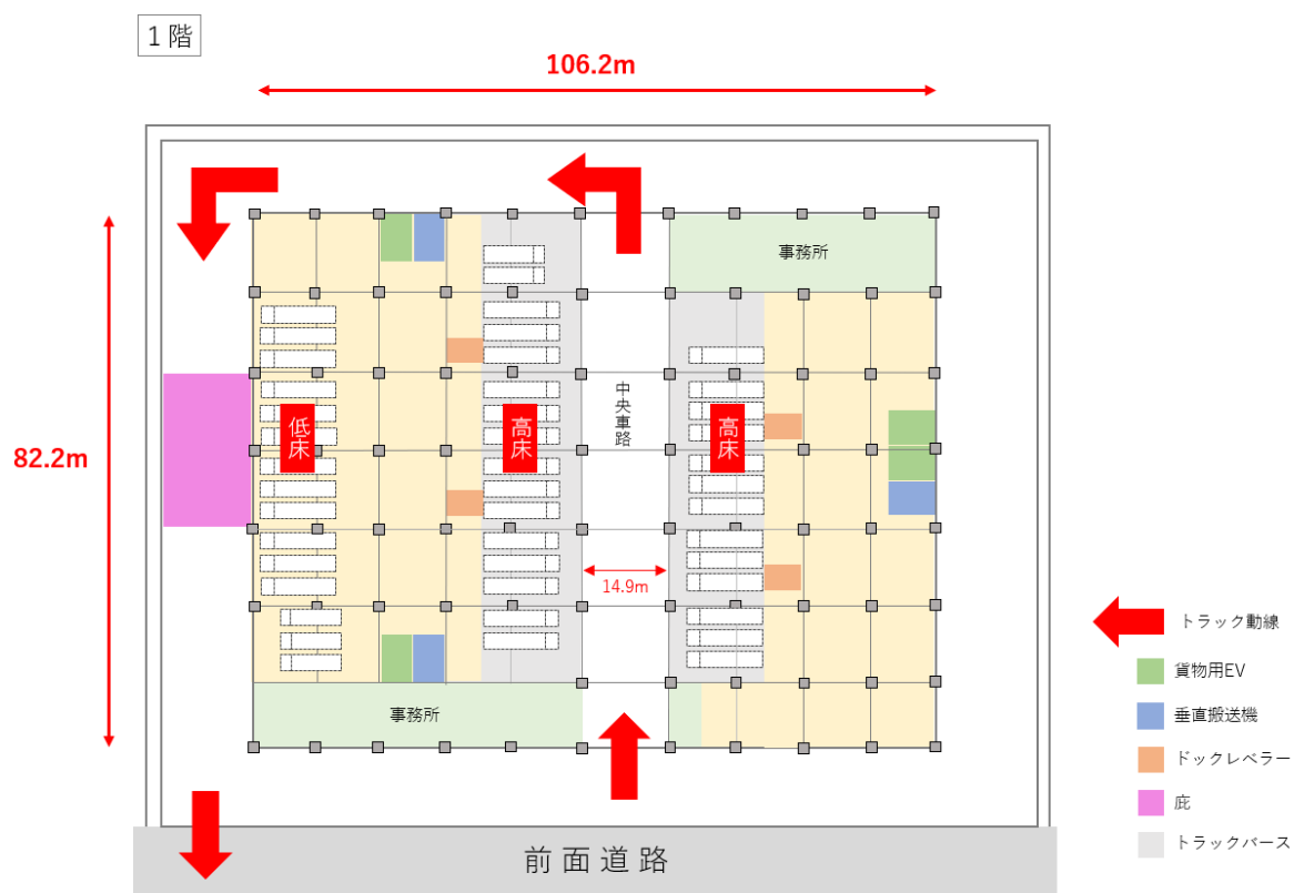
【1 階平面図】
